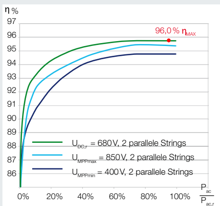
Wirkungsgradkennlinien PIKO 7.0
